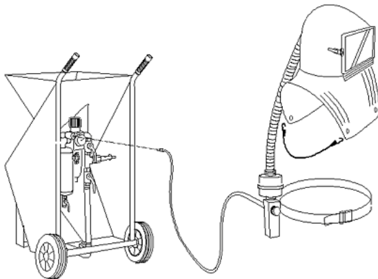
Branchement direct sur la sableuse ARENA NS10
